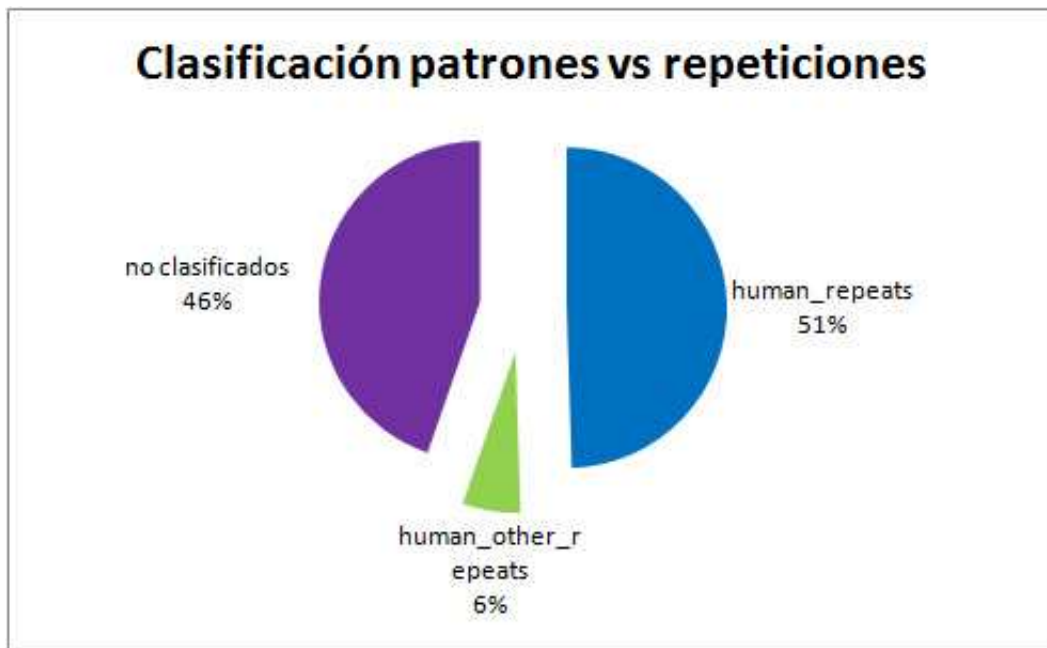
Figura 15: Patrones vs. human_repeats y human_other_repeats (solapamiento exacto) Notar que el total no suma el 100%, debido a que entre el 51% y el 6% la intersección es no vacía, como lo mencionamos anteriormente en un pie de página.
