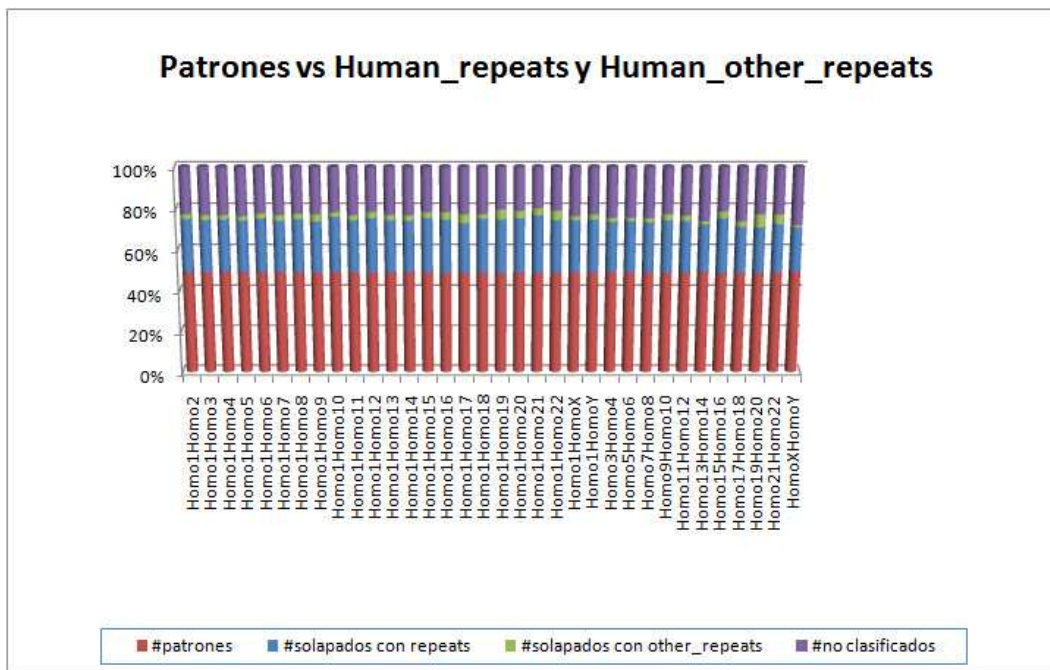
Figura 13: Patrones vs. human_repeats y human_other_repeats (solapamiento exacto) Este gráfico resume la información resultante de las comparaciones hechas bajo este criterio. Aproximadamente el 54% de los patrones fueron biológicamente identificados, y un 46% no pudo ser clasificado. Detalle de los datos para este gráfico en el apartado A.
