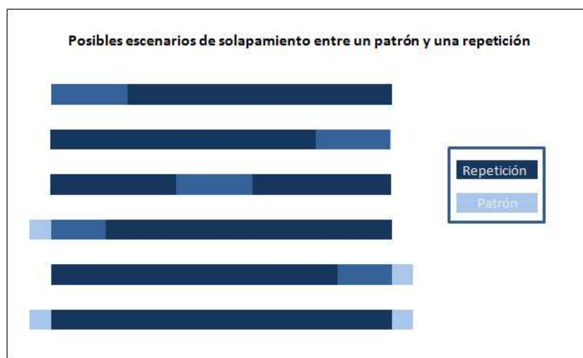
Figura 14: Los distintos casos de solapamiento entre un patrón y una repetición que pueden darse.
