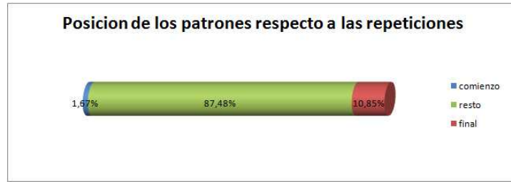
Figura 17: Posición de los patrones respecto a las repeticiones
